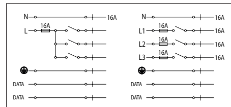
Schema elettrico Electrical scheme
